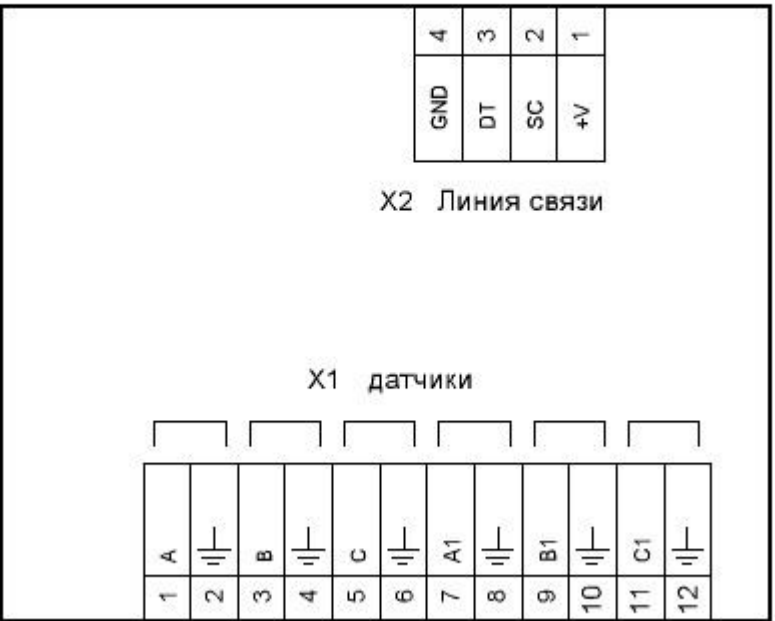
Схема подключения коммутатора СКВН2
